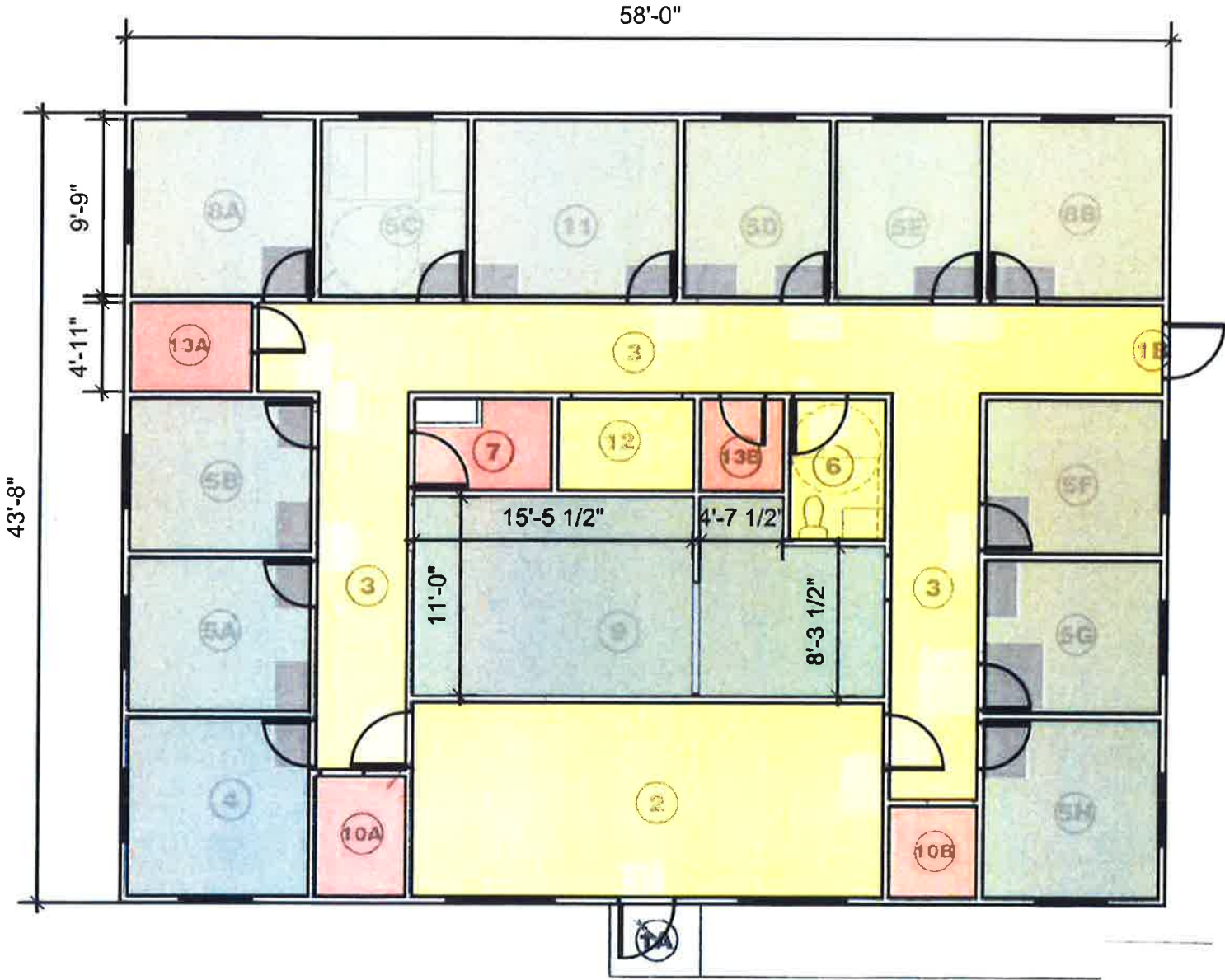
1 3306 Renner, Fortuna - Floor Plan Scale: 1/8" = 1'-0"
